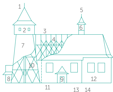
Konstrukcja gotyckiego drewnianego kościoła z dobudowaną wieżą: 1–krzyż, 2–izbica, 3–kalenica, 4–wieża dachowa, 5–krzyż, 6–sygnaturka, 7–wieża, 8 i 9–kruchta, 10–konstrukcja wieży, 11–nawa główna, 12–prezbiterium
