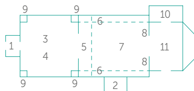
Rzut poziomy typowego gotyckiego drewnianego kościoła z dobudowaną wieżą: 1 i 2–kruchta, 3–przedśionek, 4–wieża, 5–chór muzyczny, 6–zaskrzynienia, 7–nawa główna, 8–ściana tęczowa, 9–główne słupy konstrukcji wieży, 10–zakrystia, 11–prezbiterium
