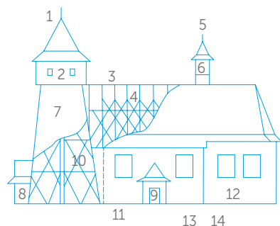
Konstrukcja gotyckiego drewnianego kościoła / cerkwi z dobudowaną wieżą: 1–krzyż, 2–izbica, 3–kalenica, 4–wieżba dachowa, 5–krzyż, 6–sygnaturka, 7–wieża, 8 i 9–kruchta, 10–konstrukcja wieży, 11–nawa główna, 12–prezbiterium
