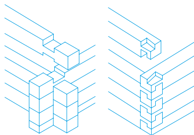
Narożnik budynku o konstrukcji zrębowej (dwa rodzaje wiązań)
