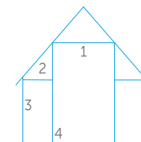
Przekrój poprzeczny kościoła / cerkwi: 1–strop, 2–zaskrzynienie, 3–obniżony zrąb nawy, 4–zrąb prezbiterium
