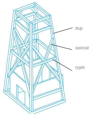
Wieża o konstrukcji szkieletowej
