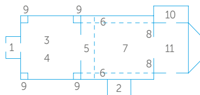
Rzut poziomy typowego gotyckiego drewnianego kościoła / cerkwi z dobudowaną wieżą: 1 i 2–kruchta, 3–przedścionek, 4–wieża, 5–chór muzyczny, 6–zaskrzynienia, 7–nawa główna, 8–ściana tęczowa, 9–główne słupy konstrukcji wieży, 10–zakrystia, 11–prezbiterium
